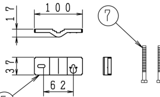
【マスト保持金具】
