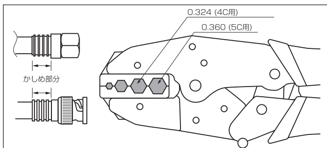
六角圧着工具 HT-RCR
