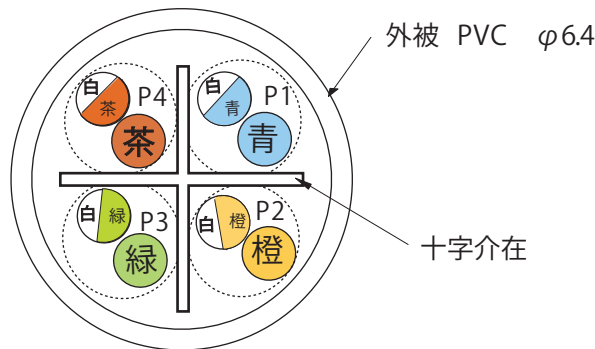
断面構造図
