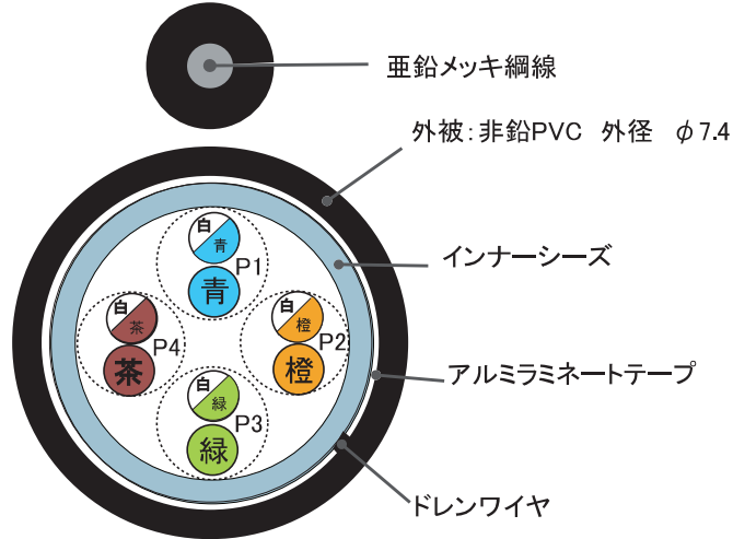
断面構造図
