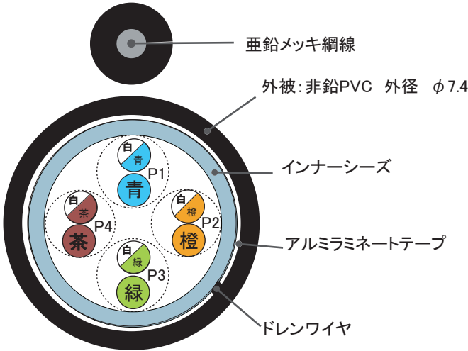
断面構造図
