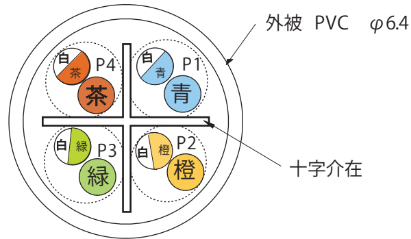
断面構造図
