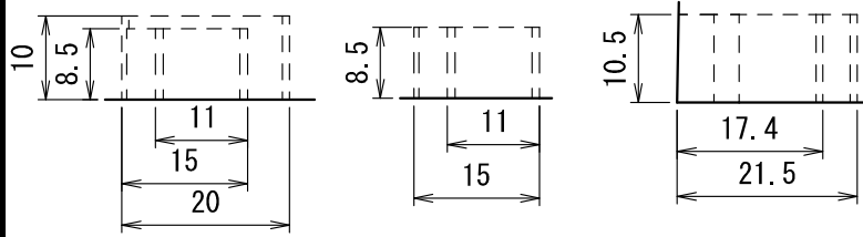
側面ロックアウト A 詳細 (1/1) 側面ロックアウト B 詳細 (1/1) 側面ロックアウト C 詳細 (1/1)
