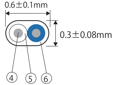
テープ心線
